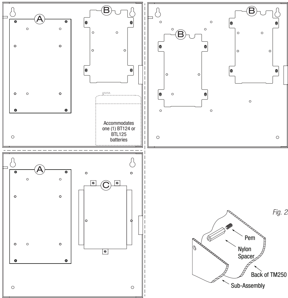
Fig. 2 - TM250 Configurations
