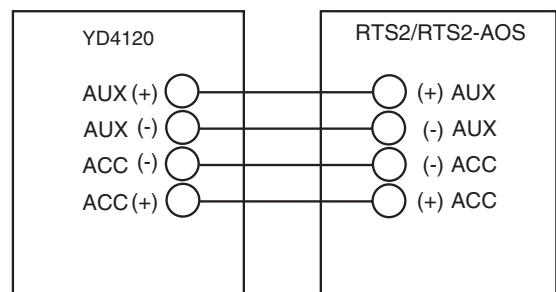
FIGURE 14. WIRING DIAGRAM FOR D4120 TO RTS2/RTS2-AOS:
